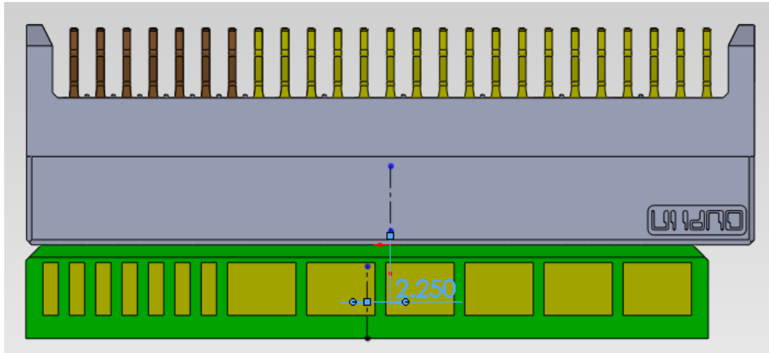
allowed misalignment in transverse axes 在橫向方向允許對插偏差量
