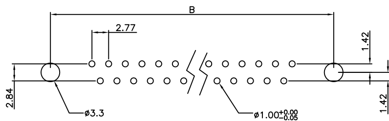
P.C.Board Layout
