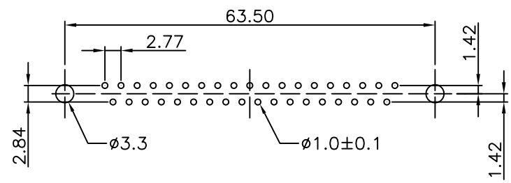
P.C.Board Layout
