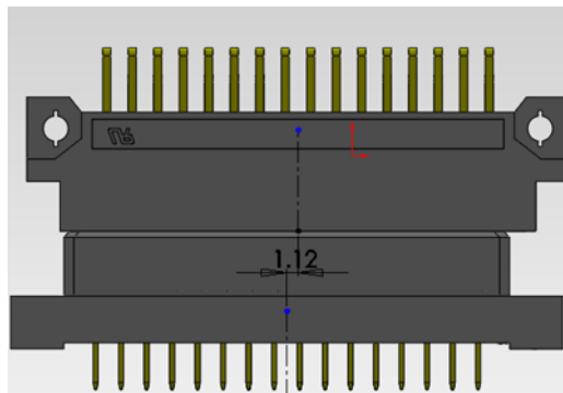
allowed misalignment in longitudinal axes 在縱向方向允許對插偏差量
