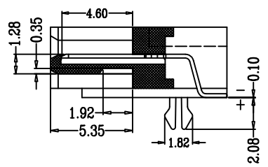
Sect A-A
