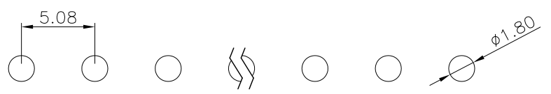
P.C.Board Layout
