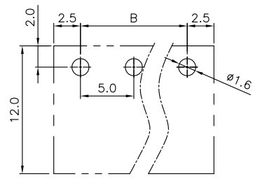
P.C.Board Layout
