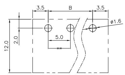
P.C.Board Layout
